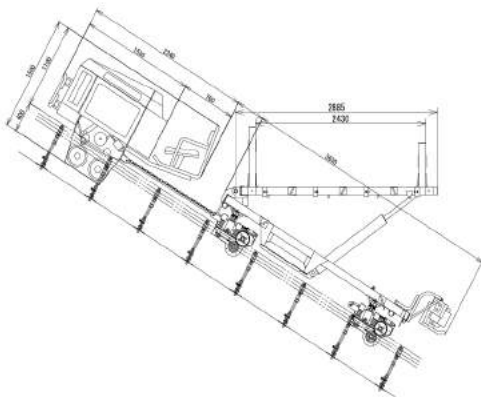
動力車 KS-400+ リフター台車
