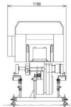
動力車 KS-400
