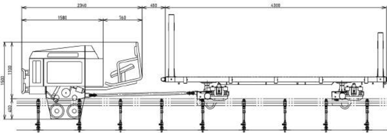
動力車 KS-400+ リフター台車
